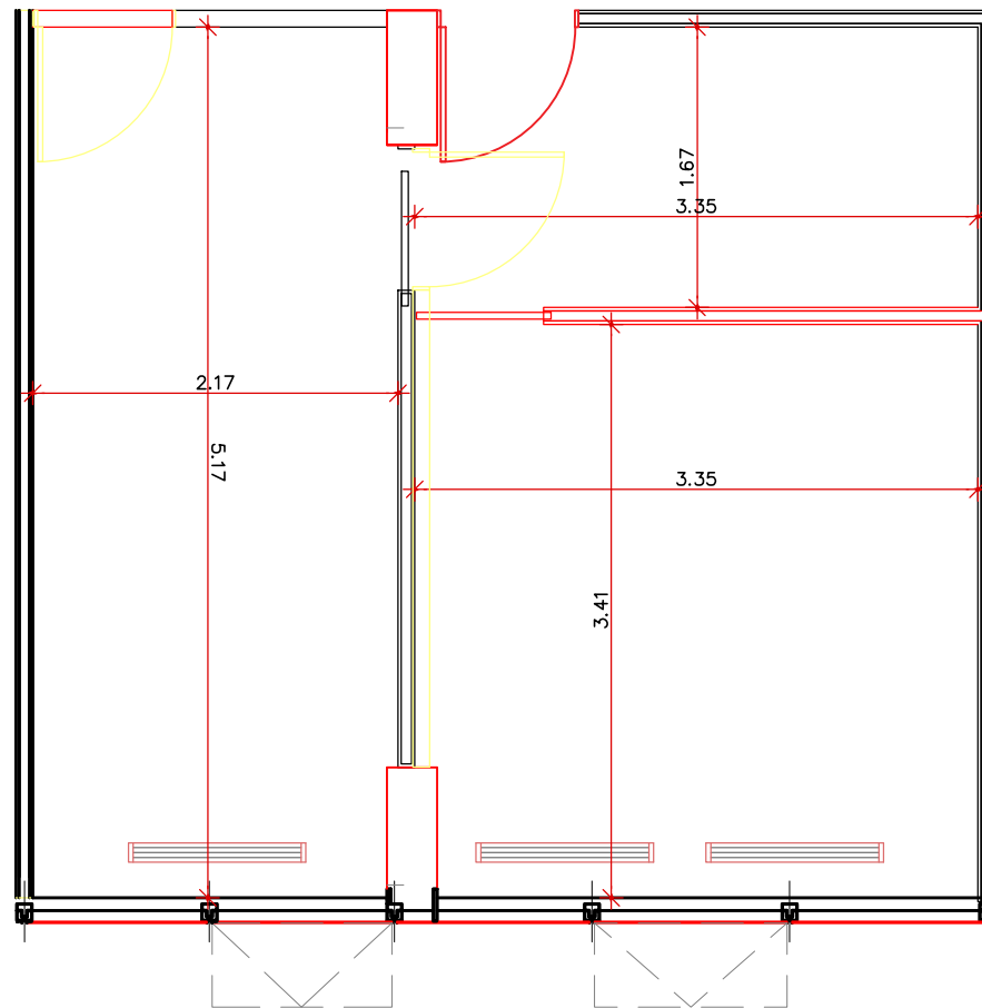
MOVIMENTAÇÃO DE PAREDES/ DIVISÓRIAS PROPOSTA 2 ESCALA 1:50
