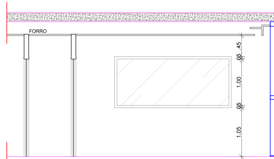
CORTE AA-Elevação ESCALA ..... 1/50
