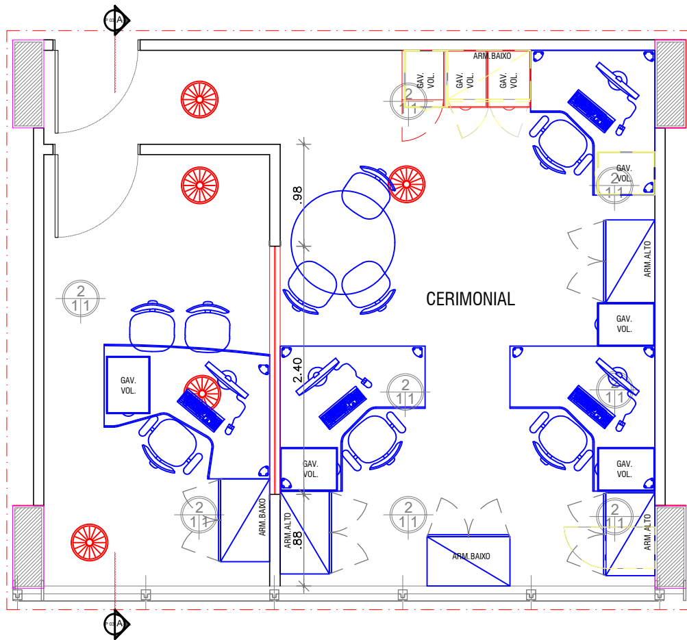
PLANTA BAIXA Nova proposta
