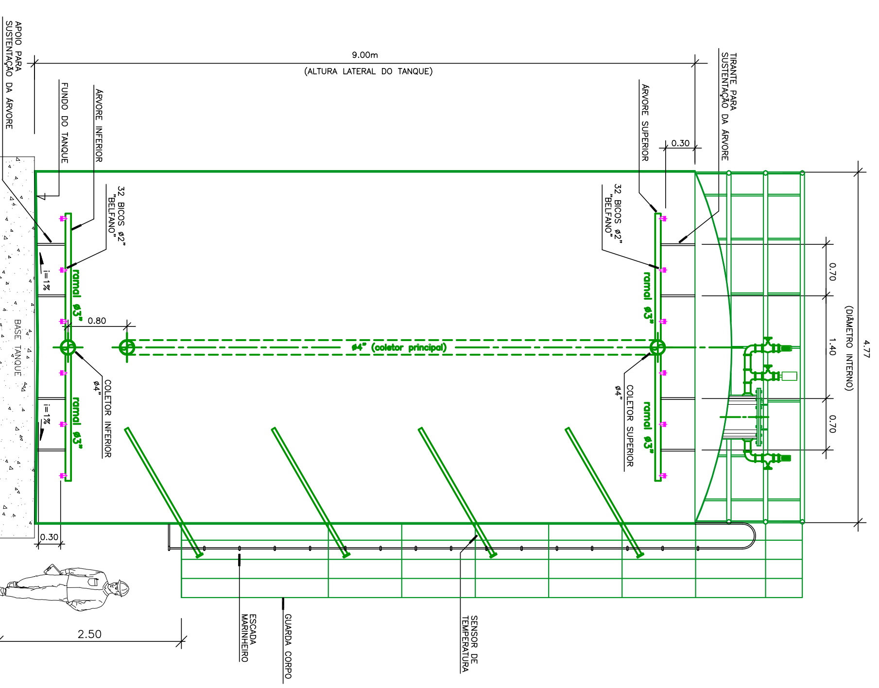
CORTE AA ESCALA 1/20
