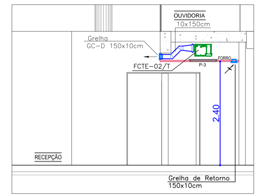
CORTE DET. 2 - TÉRREO ESCALA 1/30
